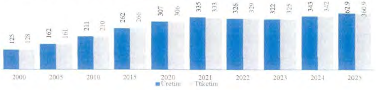
Grafik: Türkiye'nin Elektrik Üretiminin ve Tüketiminin Gelişimi (TWh)
