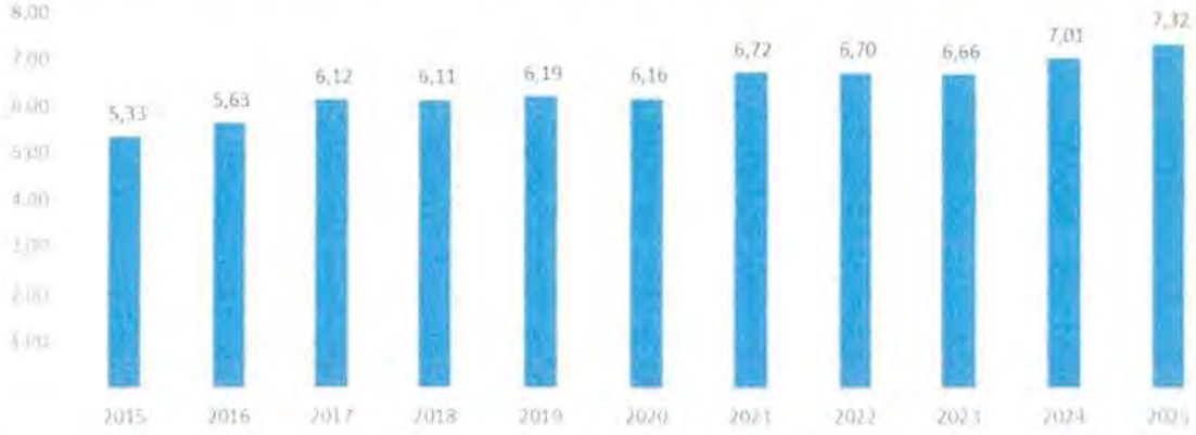
Grafik: 2015 ve 2025 Yılları Arasında Türkiye Enerji Tüketiminin Gelişimi (EJ)
